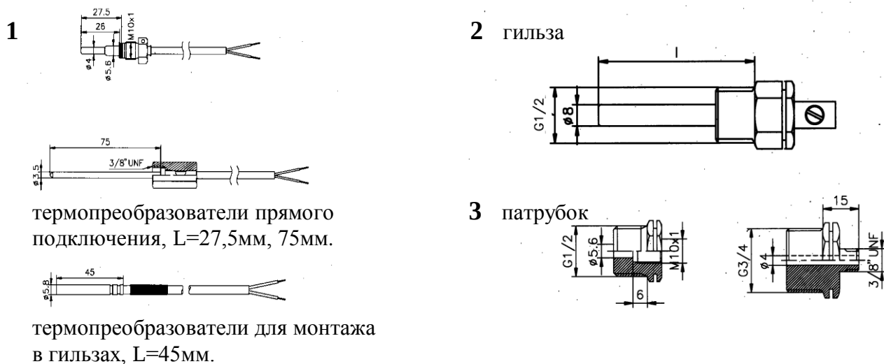
Рис. 2. Термопреобразователи сопротивления.
