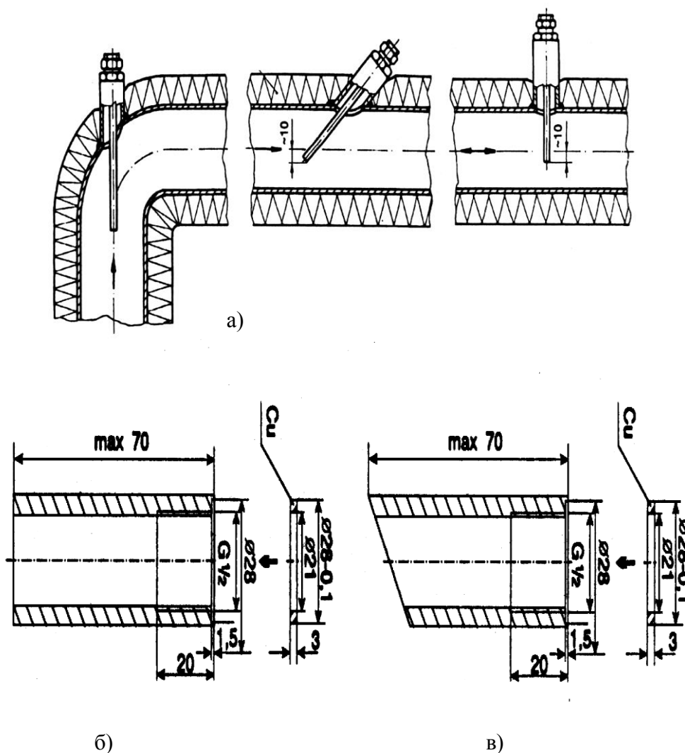
Рис. 3. Монтаж термopеобpазователей сопротивления.
