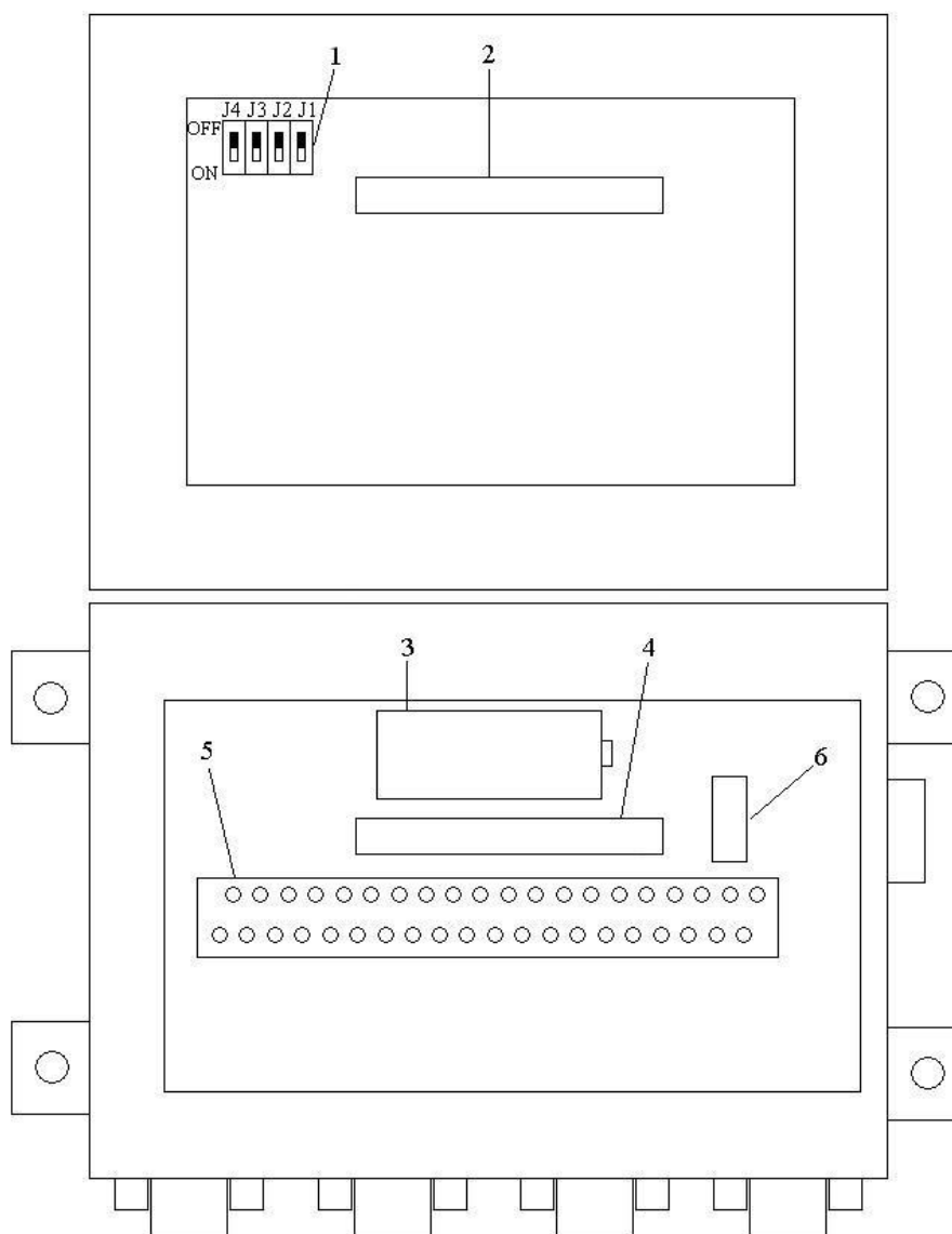
Рис.5. Вид тепловычислителя с открытой верхней крышкой.
