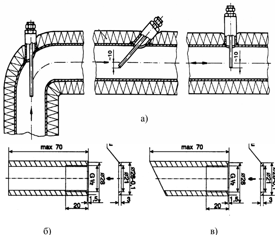
Рис. 3. Монтаж термопреобразователей сопротивления.
