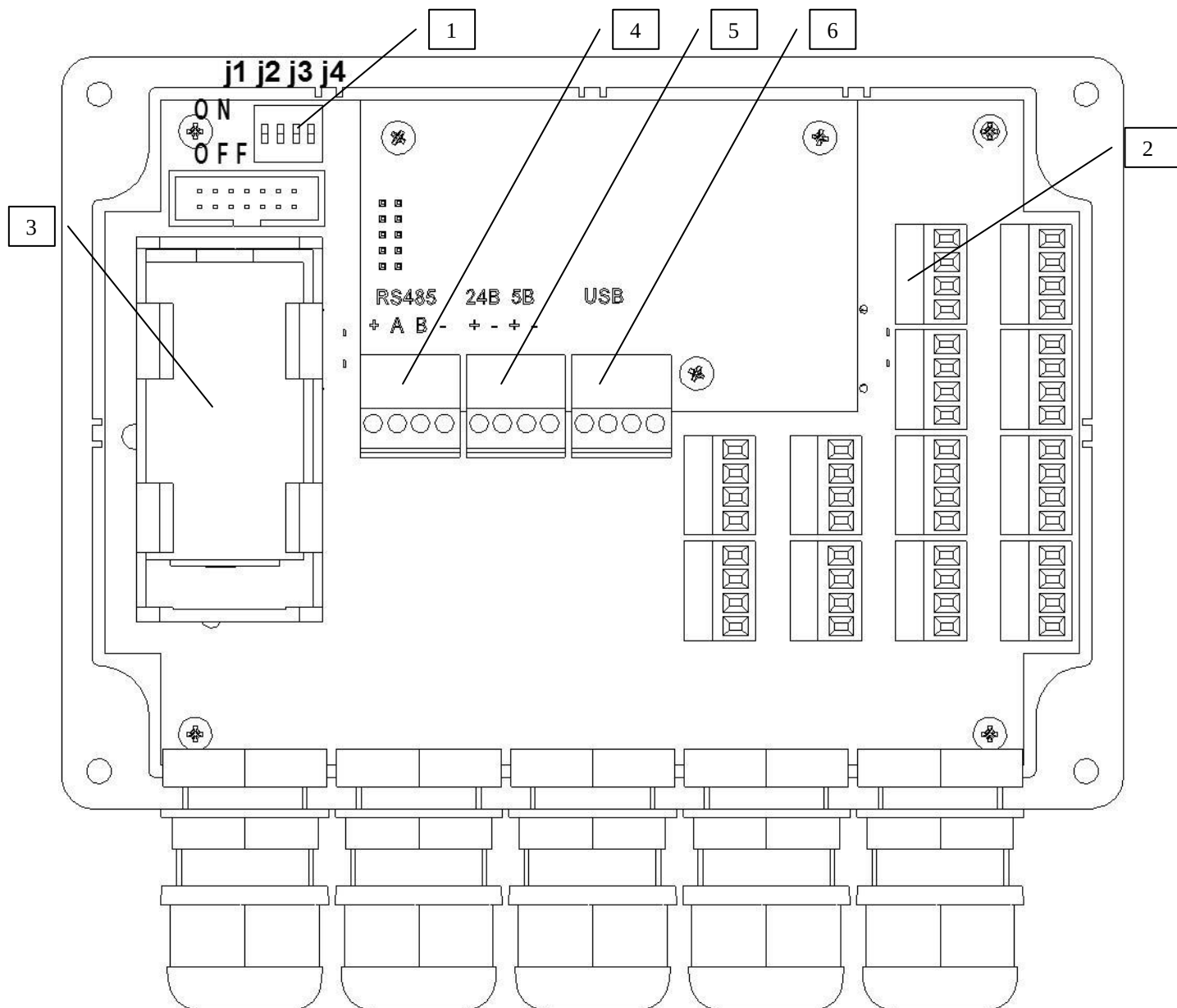
Рис. 6. Вид тепловычислителя ВТЭ-ІІІ М
